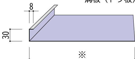
片折れ板（ケラバ用）
